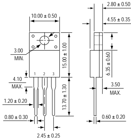
ITO-220AB
