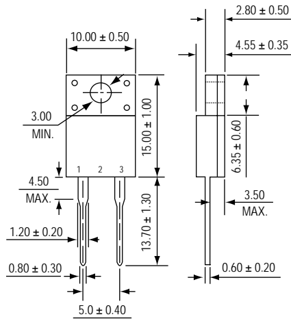
ITO-220AC
