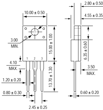
ITO-220AB
