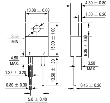
TO-220AC
