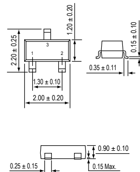
SOT-323
