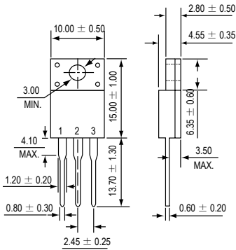
ITO-220AB
