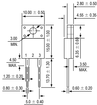
ITO-220AC
